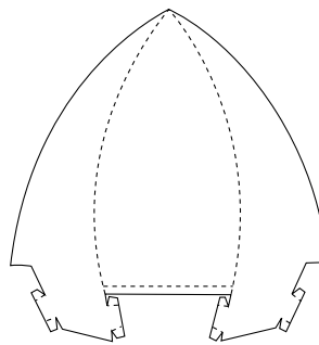
7 lampskärmsenheter 2
