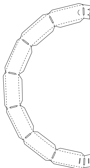
1 ringelement M
