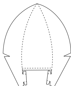
7 elementi paralume n. 1
