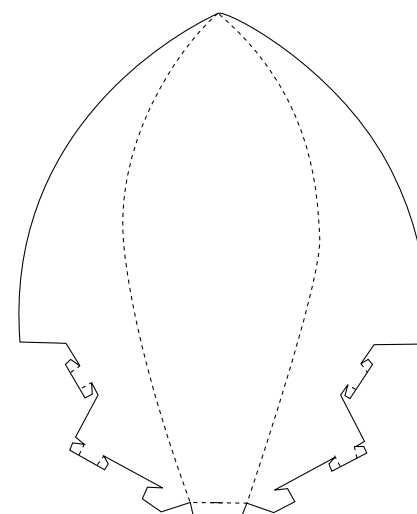
7 abat-jour n°3
