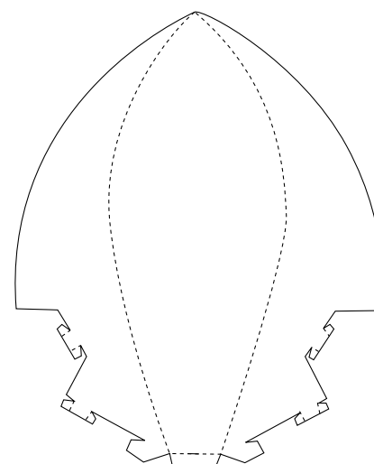
7 elementi paralume n. 3
