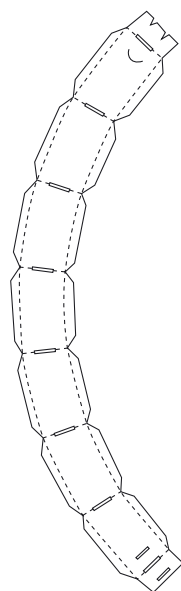
1 ringelement S
