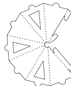
1 opphengingsmodul
