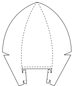
7 elementos do abajur n.º 1
