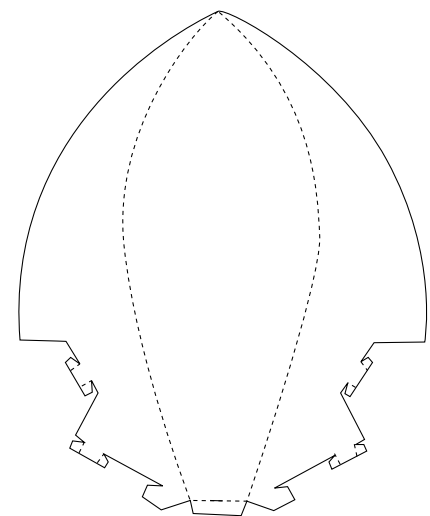
7 lampenkap-elementen nr. 3
