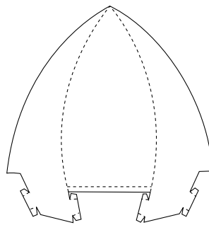
2번 전등갓 구성요소 7개
