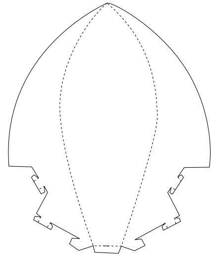
3번 전등갓 구성요소 7개
